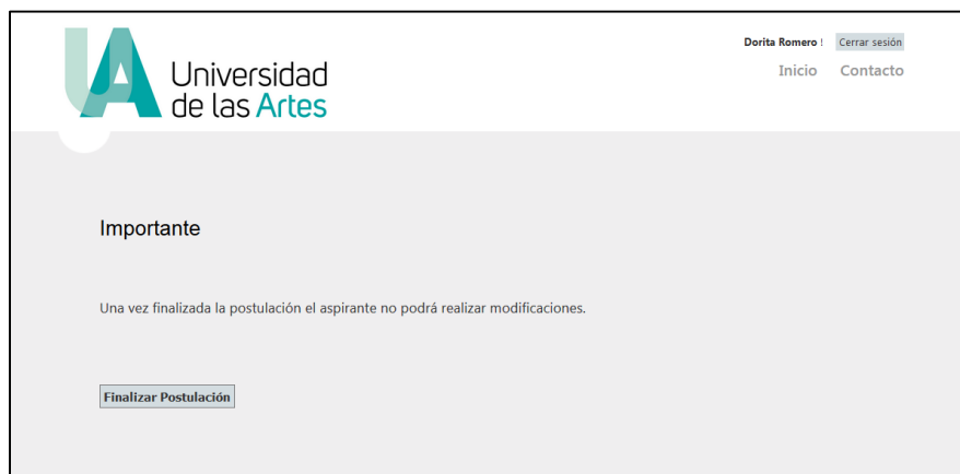
Figura 9 – Finalizar Postulación
